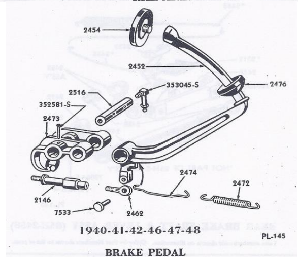
BRAKE PEDAL
